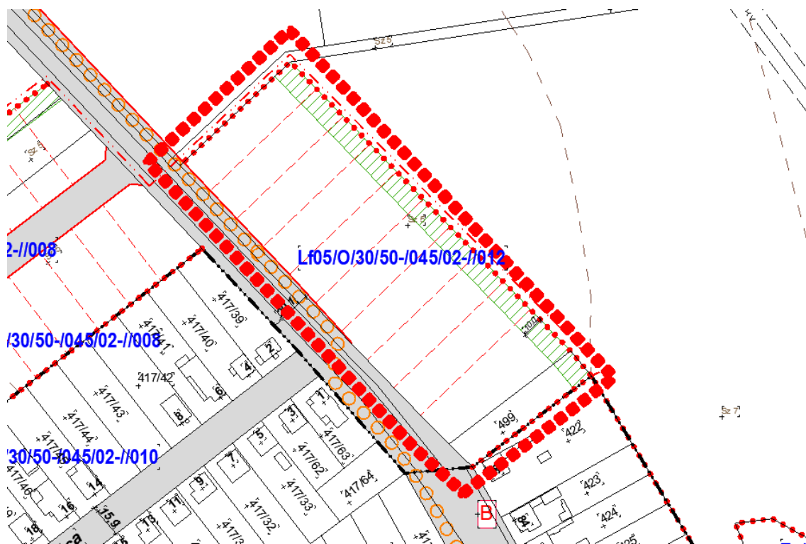
Szabályozási terv kivonat
